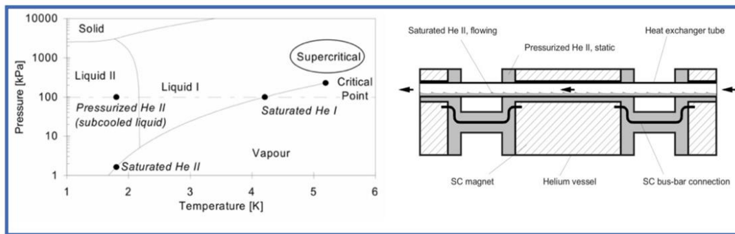
Fig. 23-8: The LHC cryogeny 669 .
